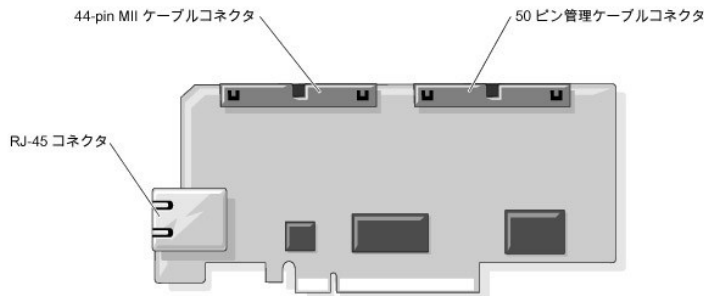
図 1-1. DRAC 5 ハードウェア機能
